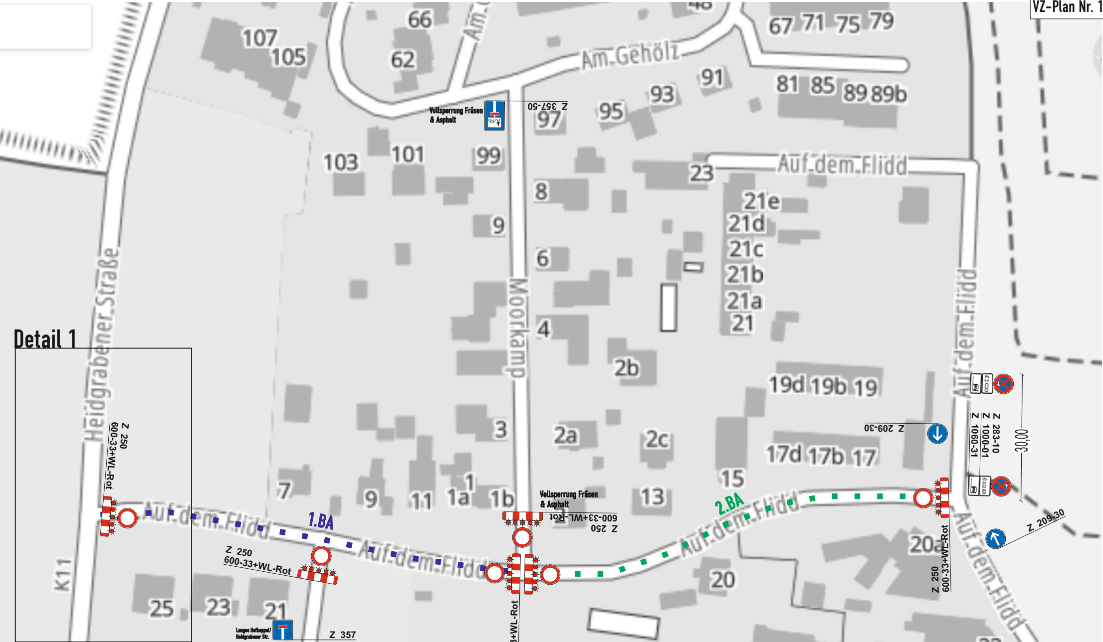
Detail 1 Fräsen & Asphalt
